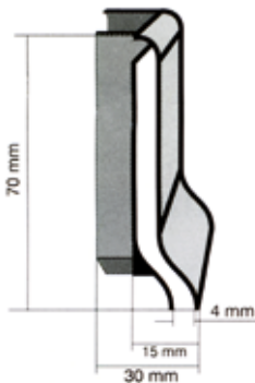
Angolare esterno
