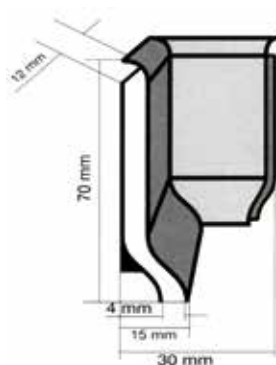
Angolare interno
